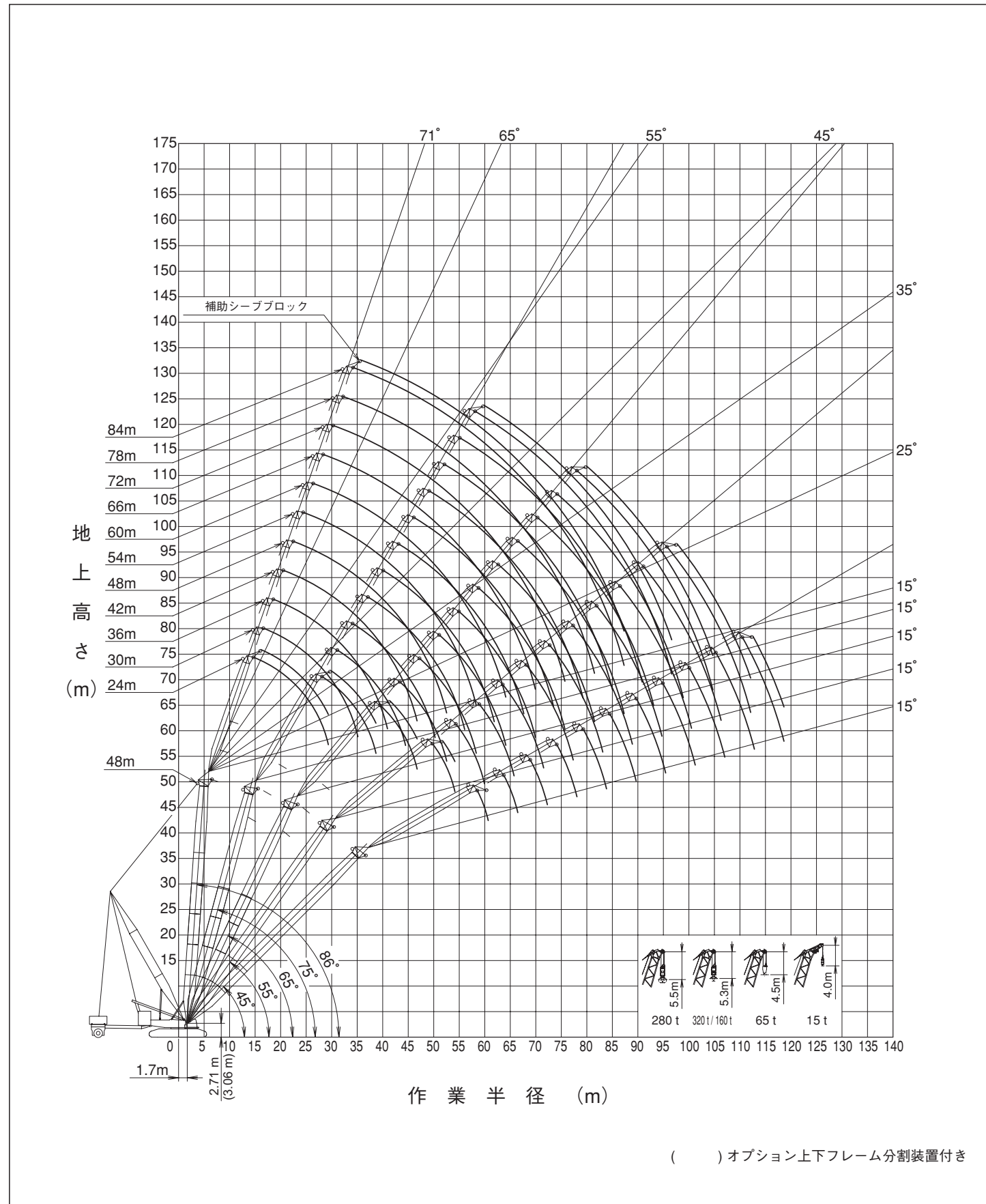
■ 作業範囲図：48 m タワー+ジブ
